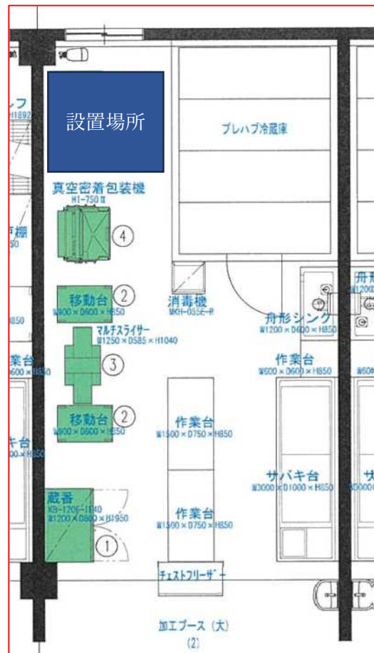
レイアウト案
